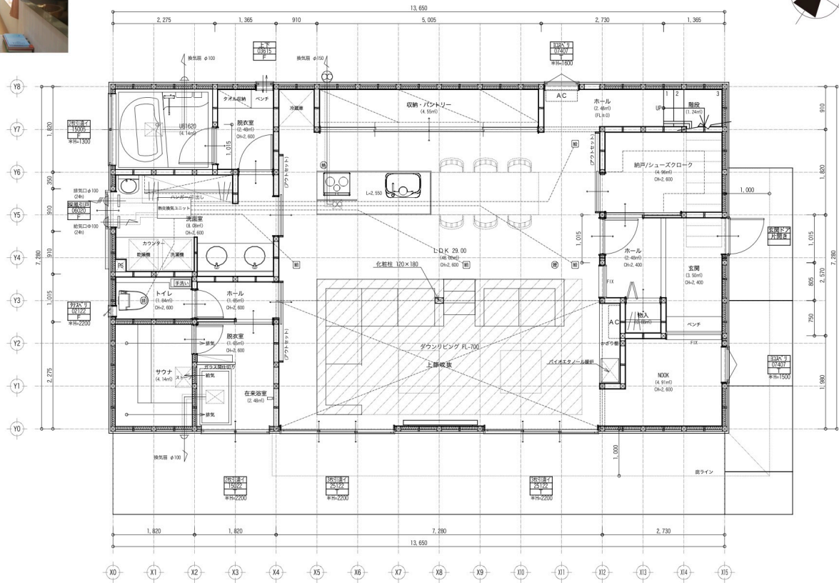
1階 平面詳細図 S:1/60
