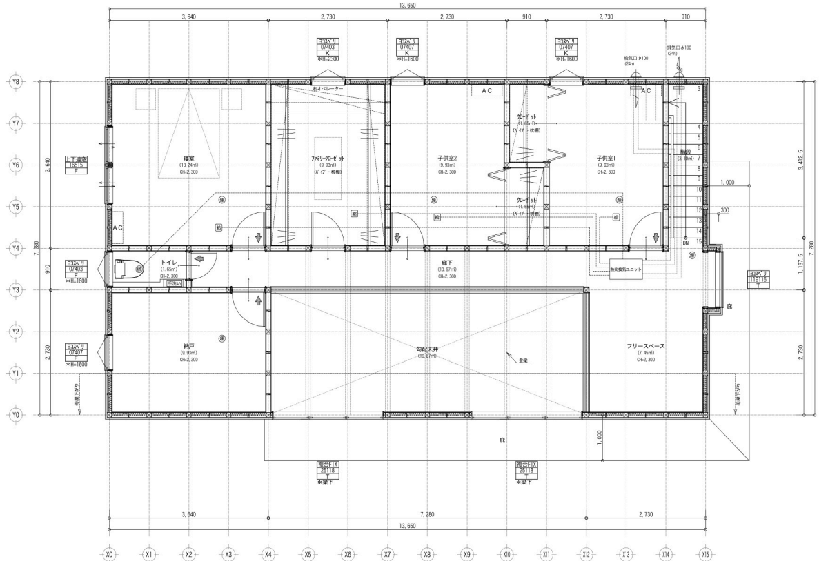
2階 平面詳細図 S:1/60
