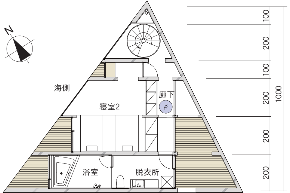
3階平面図
