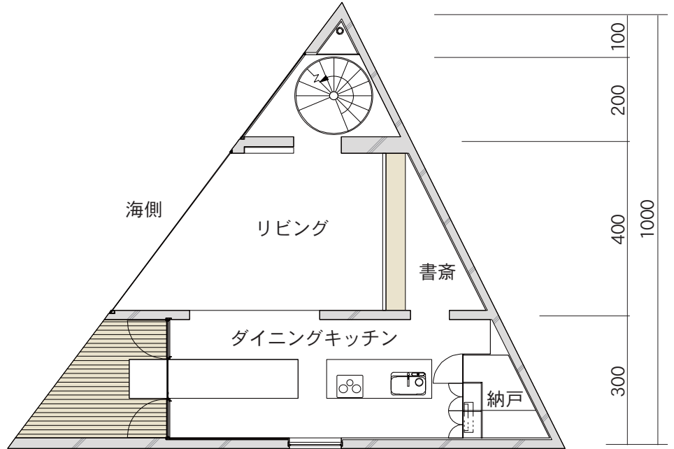
2階平面図
